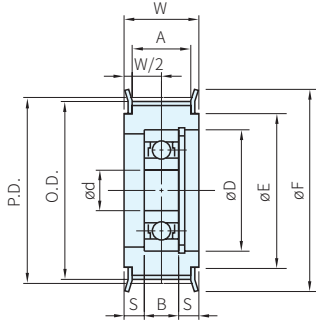
中心軸承型 (1PCS軸承時)
